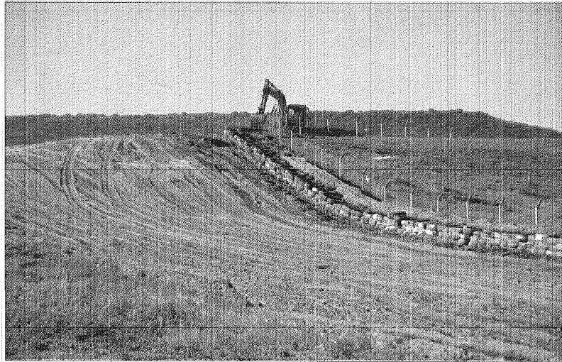
En la "trepada de Mottino", se está trabajando en las vías de escape, y asegurando los neumáticos de contención con un talud posterior.
